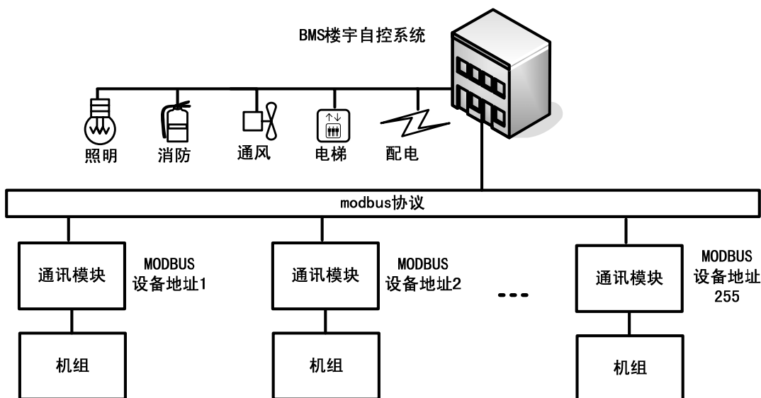
图一：拓扑图
